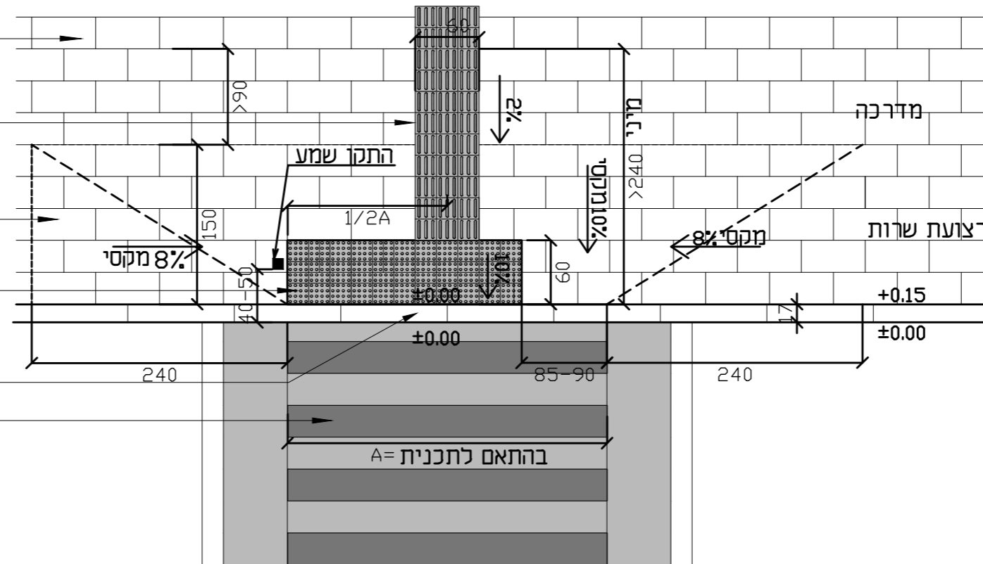
תכנית קנ"מ 1 : 50
