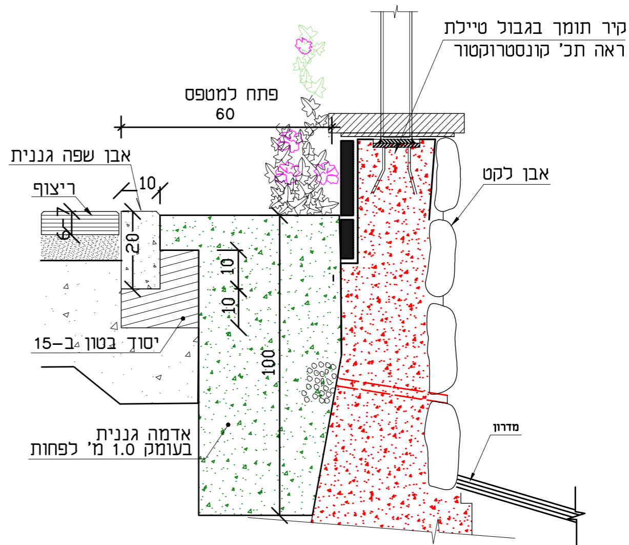
חתך אופייני על קרקע 1:10
