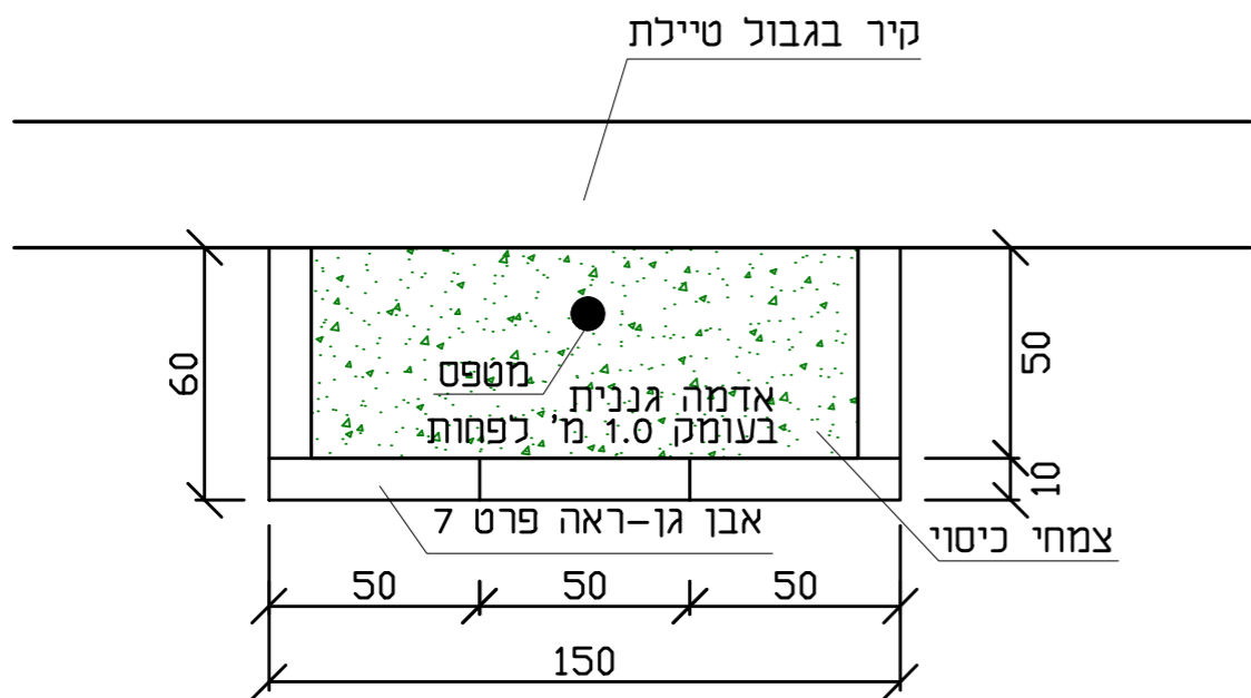
מבט על 1:20
